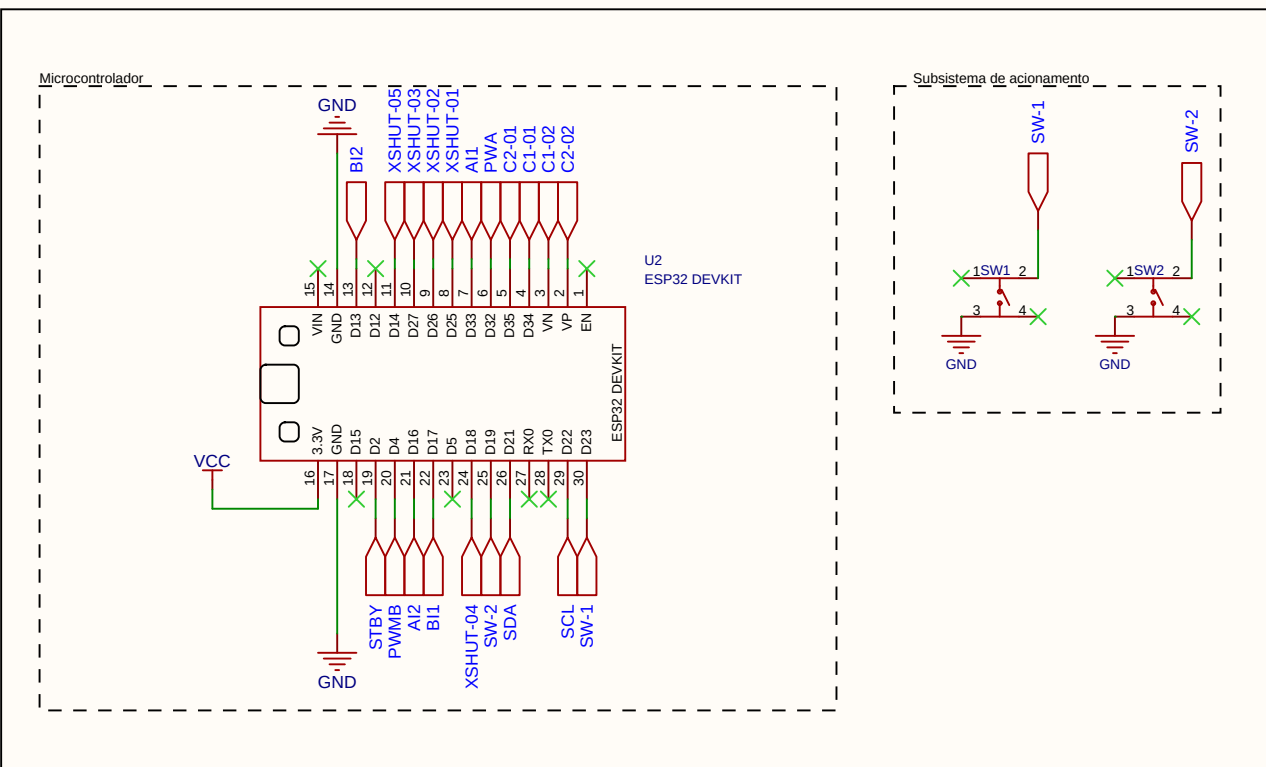
Sistema de Processamento Central
