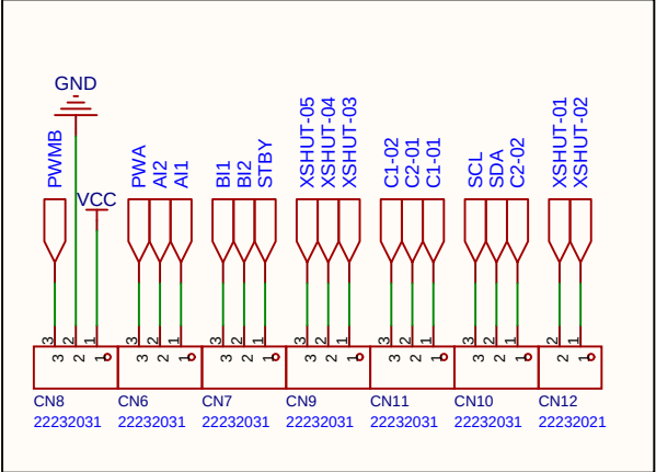
Sistemas de conexões externas
