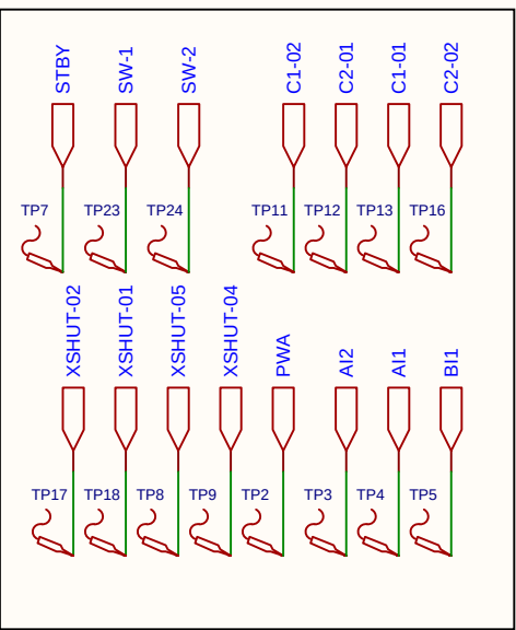
Conexões Test point
