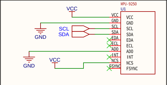
Subsistema de Navegação Inercial
